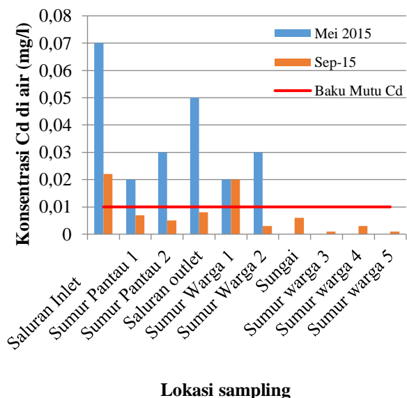
Gambar 2. Sebaran logam berat Cd di area TPA
