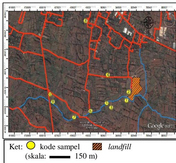
Gambar 1. Lokasi pengambilan sampel air (Peta diolah dari google earth)
