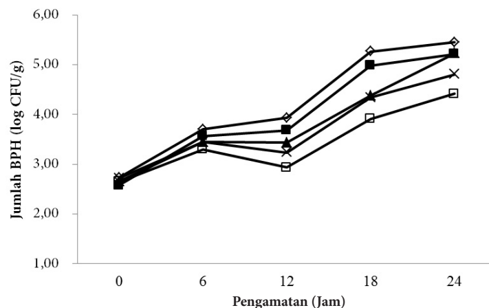
Gambar 3 Pengaruh konsentrasi ekstrak etanolik Padina sp. terhadap jumlah bakteri pembentuk histamin (BPH) ikan kembung yang disimpan pada suhu kamar (◇=0; ■=0,5; ▲=1; x=1,5; dan □=2 g/100 mL).
