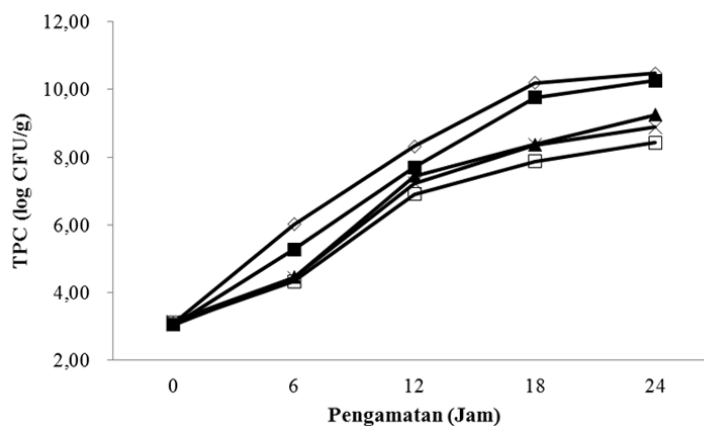
Gambar 2 Pengaruh konsentrasi ekstrak etanolik Padina sp. terhadap jumlah bakteri total (TPC) filet ikan kembung yang disimpan pada suhu kamar (◇=0; ■=0,5; ▲=1; ×=1,5; dan □=2 g/100 mL).
