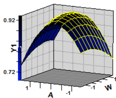
Gambar 7 Respon permukaan hubungan antara waktu sonikasi dan amplitudo terhadap stabilitas suspensi
