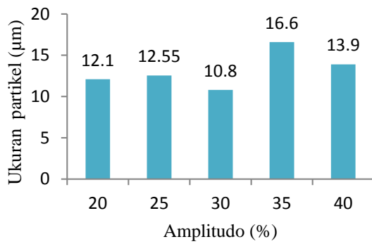
Gambar 3 Hubungan amplitudo dengan ukuran partikel pada waktu sonikasi 50 menit
